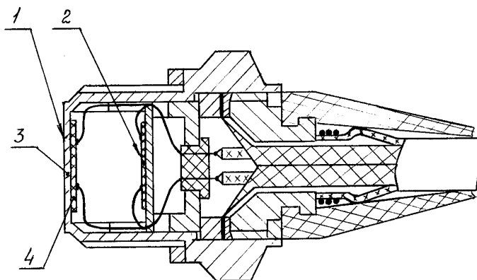
1. Рабочий ЧЭ. 2. Виброкомпенсирующий ЧЭ. 3. Мембрана. 4. Пьезоэлемент. Рис. 1. Конструкция датчика акустических давлений
