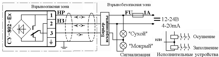
СУ взрывозащищенного Ех-Д исполнения с барьером искрозащиты
