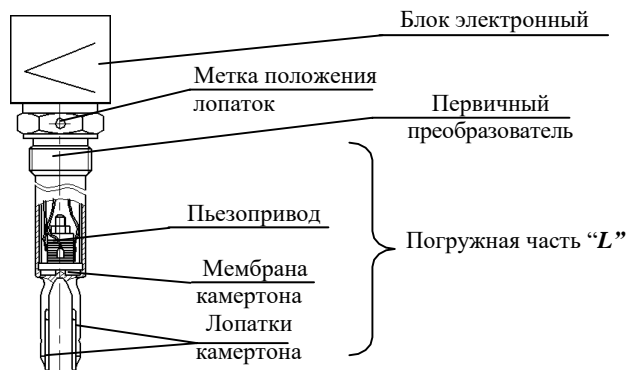
Рисунок 2 – Схема СУ
