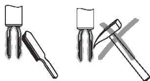
Рисунок 12 – очистка камертона
