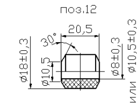
Кольца уплотнительные (варианты)
