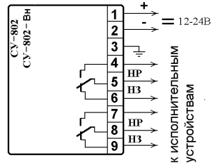
СУ взрывозащищенного Ex-N исполнения
