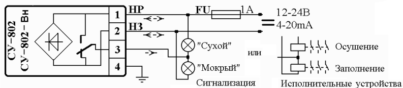
СУ обычного и взрывозащищенного Вн-Д исполнения
